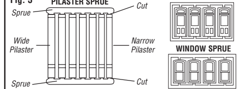
Fig. 3 PILASTER SPRUE
